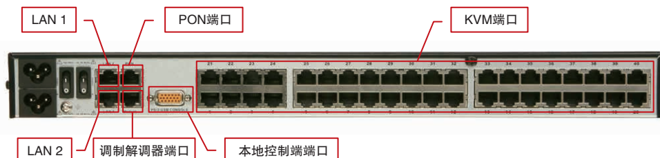
• KN2140v 后视图
