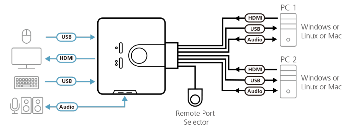
拓扑图
