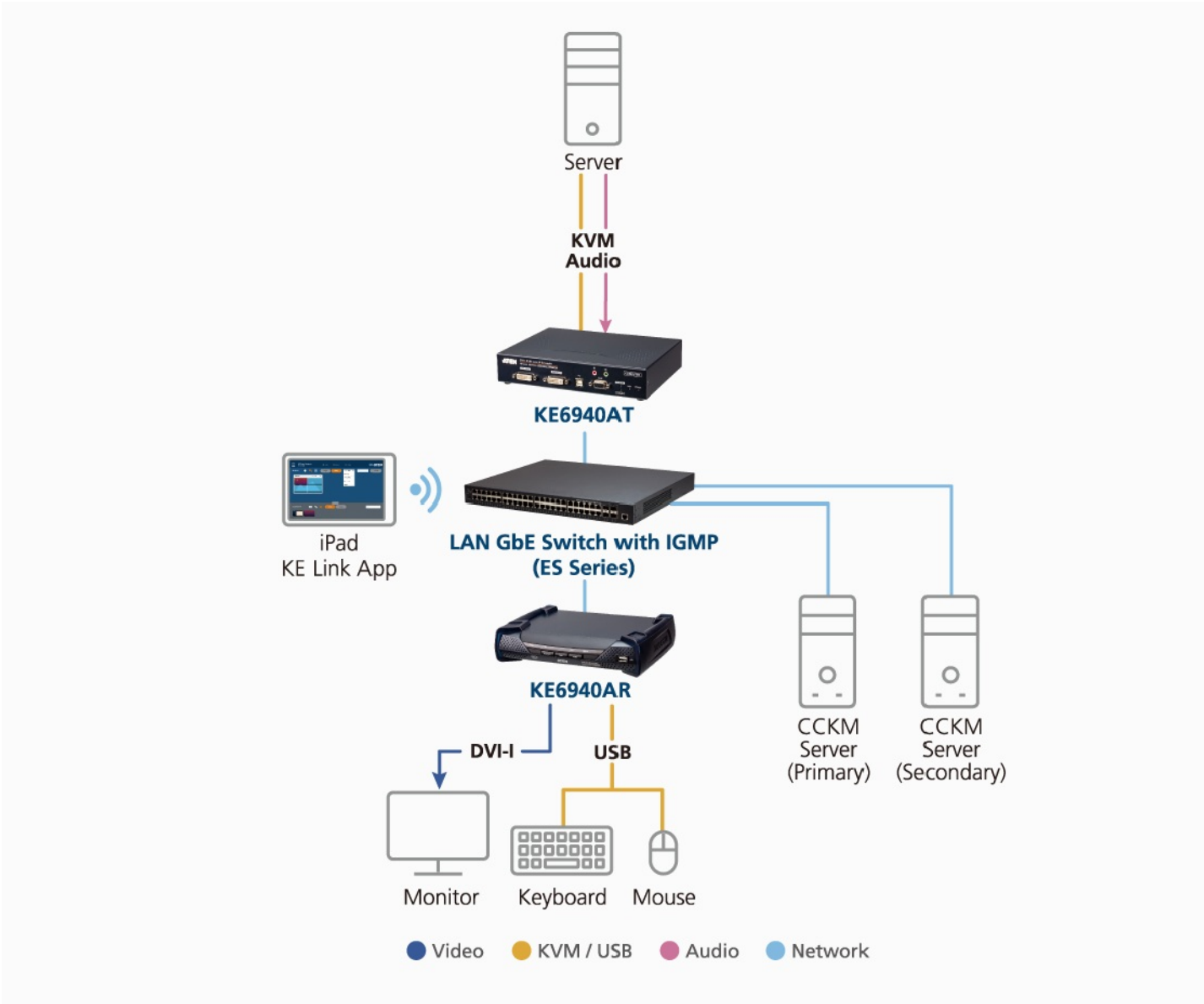
拓朴图
