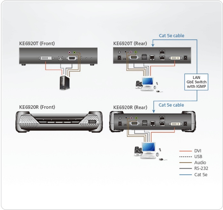
拓扑图
