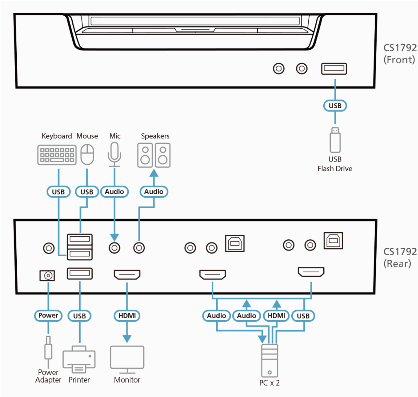
拓朴图
