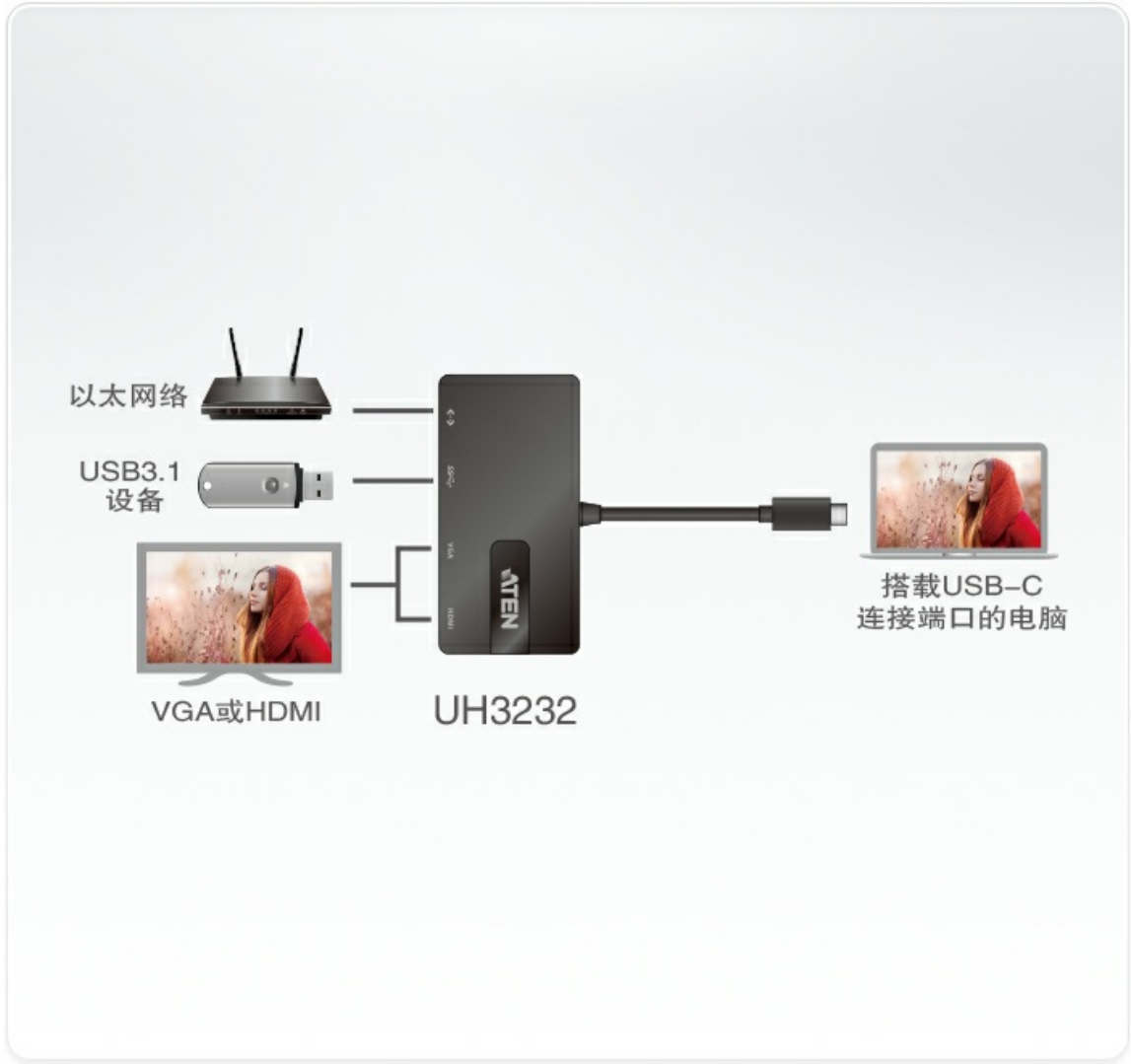
拓朴图
